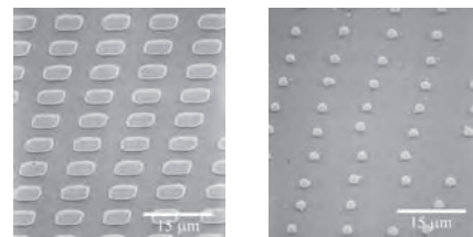
(a) レーザー照射前、(b) レーザー照射後 パルスレーザー加熱によるGe薄膜の粒子化、
