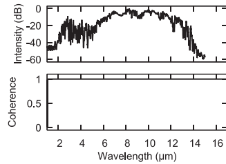
高コヒーレント中赤外スーパーコンティニューム光の特性
