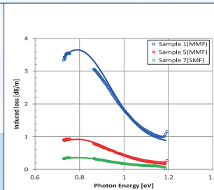
衛星間光通信用ファイバアンプの欠陥生成抑制に成功
