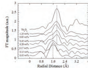
EXAFSによるシリカガラス中のYb周辺局所構造解析例
